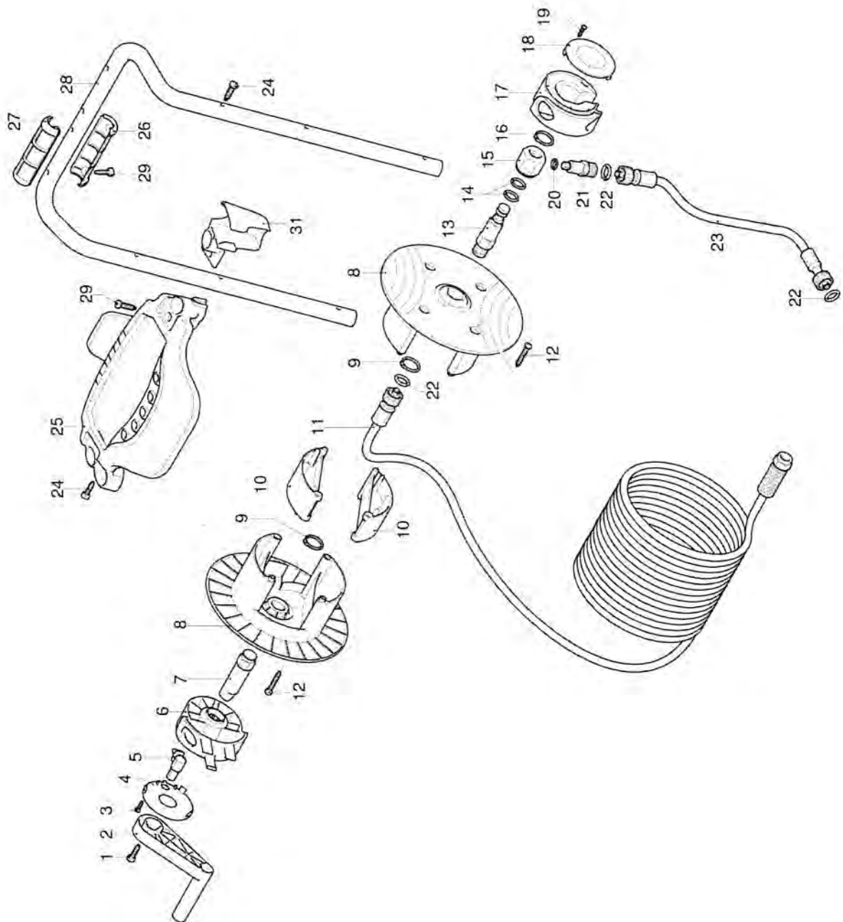
Abb. 16: Ersatzteilzeichnung 6
