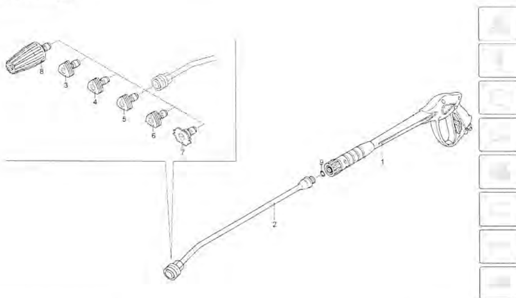
Abb. 15: Ersatzteilzeichnungen 4 und 5
