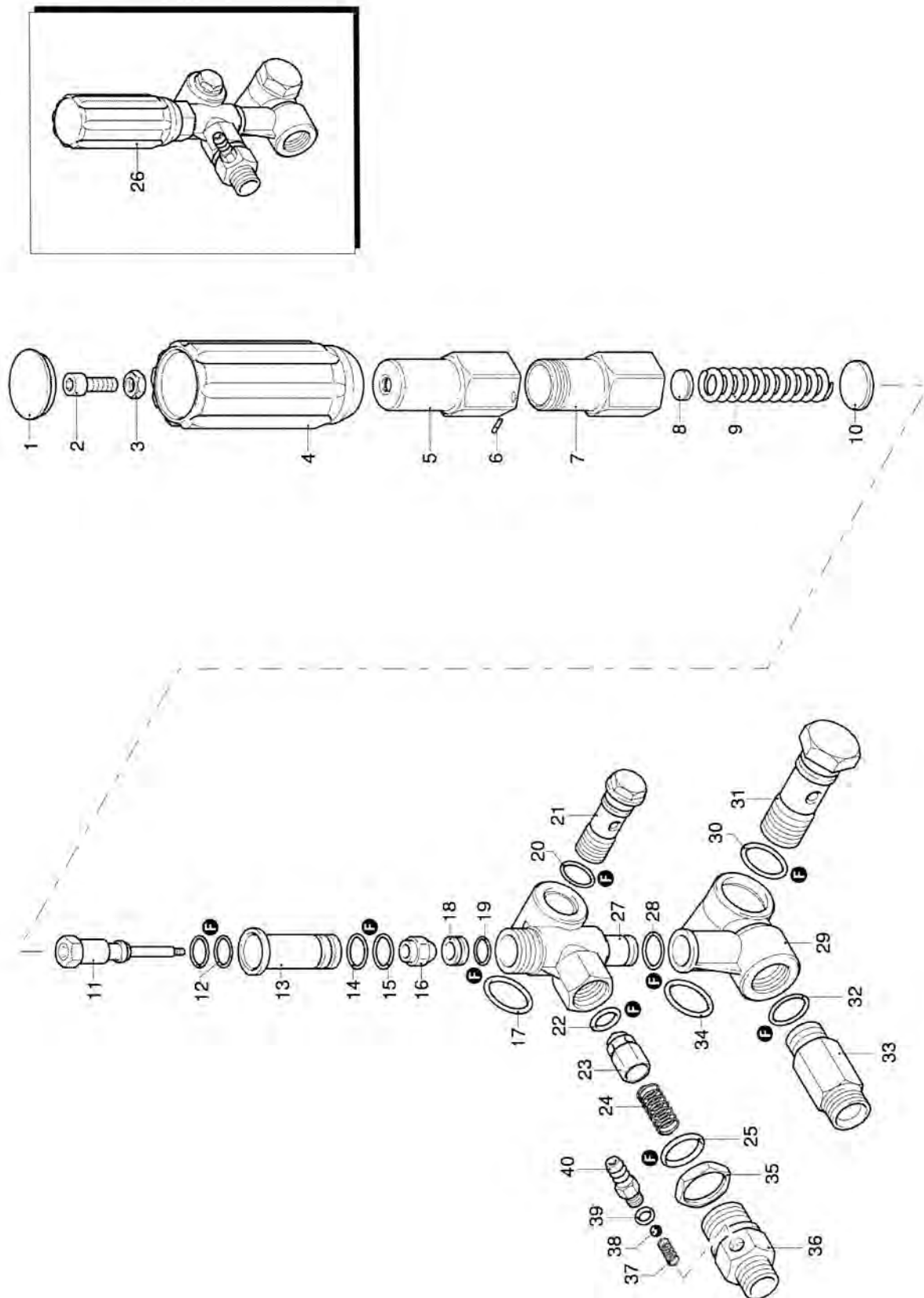
Abb. 14: Ersatzteilzeichnung 3
