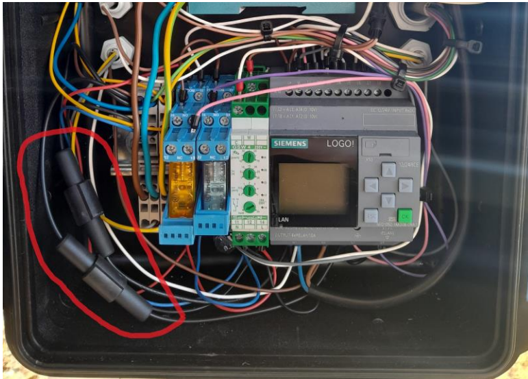
Bild 5: Sicherungshalter Schwarz für die Feinsicherung im Gerätekoﬀer
